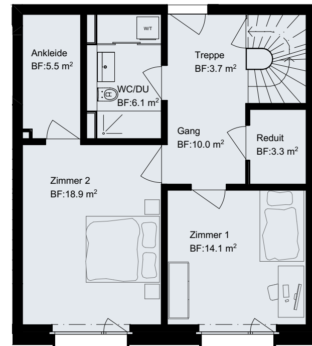
1. OG
