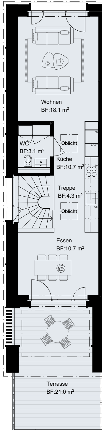
2. OG Dachgeschoss
